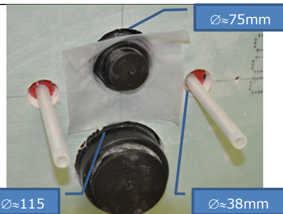
2b. Hulldimensjoner
