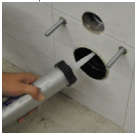
8b. Fyll også overgangen mellom avløpsbendet og resten av beskyttelsestersen med tettmassen.
